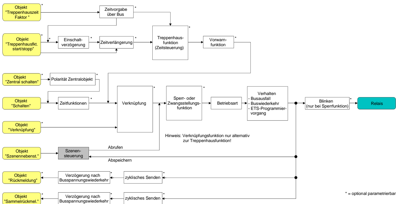
Bild 15: Funktionsschaltbild der Szenenfunktion
