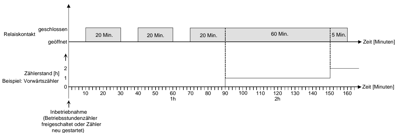
Bild 16: Funktionsweise des Betriebsstundenzählers
