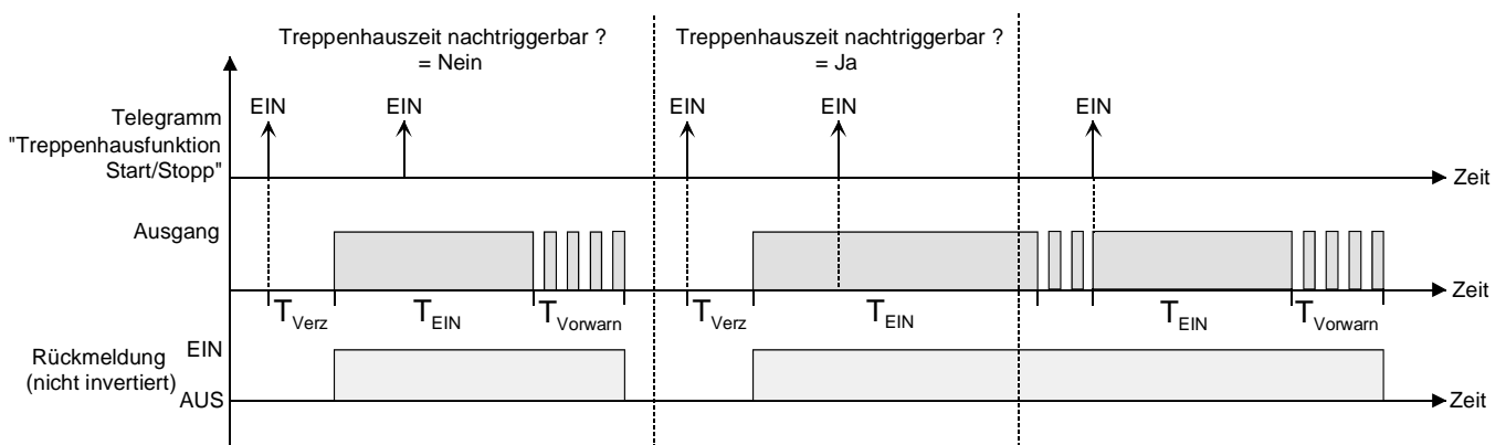
Bild 11: Einschaltverhalten der Treppenhausfunktion
