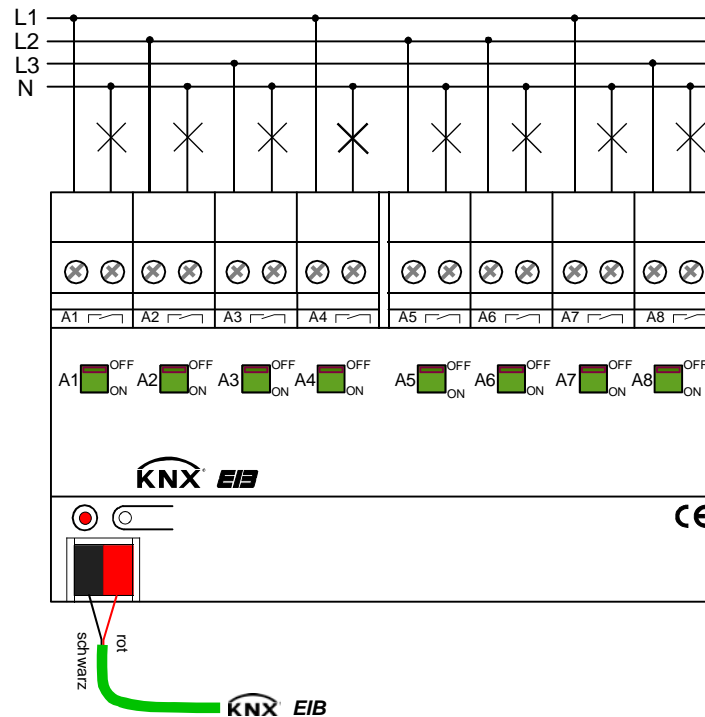
Bild 1: Elektrischer Anschluss
