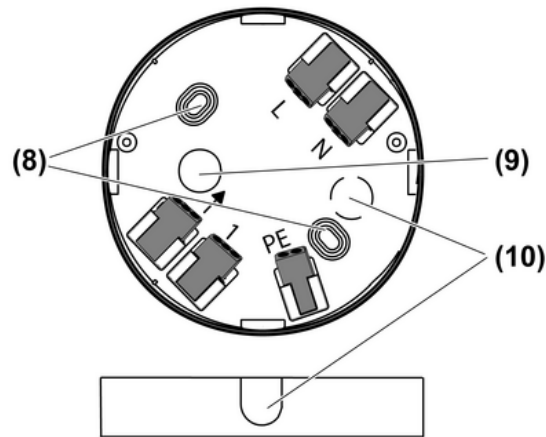
Imagen 5: Caja de conexiones
