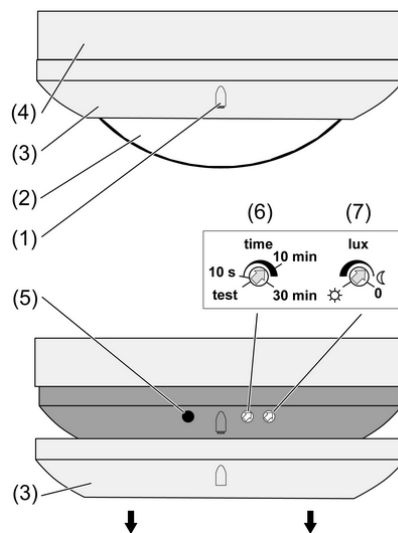
Imagen 1: Estructura del mecanismo
