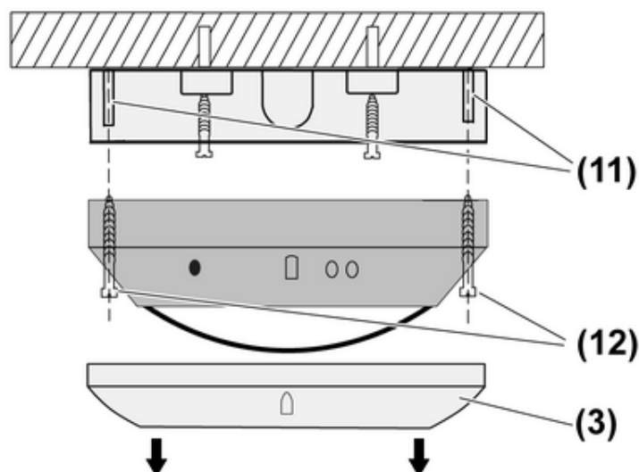
Imagen 4: Montaje
