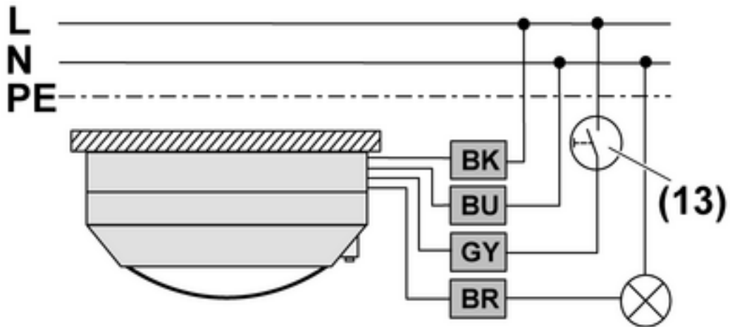
Imagen 6: Plano de conexión
