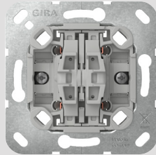
Wipdrukcontact 4-voudig (met klauwen) Artikelnr. 3147 00
