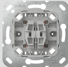
Wipdrukcontact 2-voudig (zonder klauwen) Artikelnr. 3875 00
