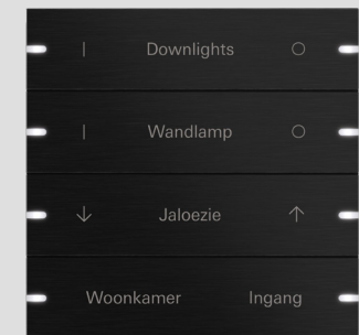
Tastsensor 4.95, 24 V 4-voudig
