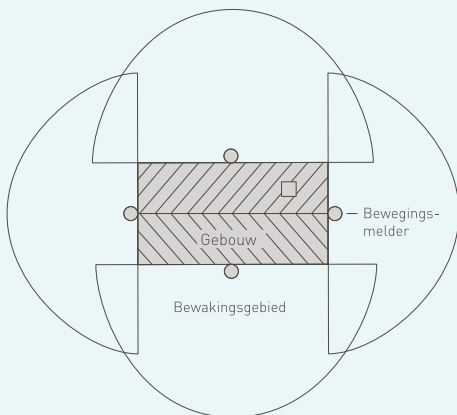
Omvangrijk bewakingsgebied bestaande uit vier eNet bewegingsmelders
