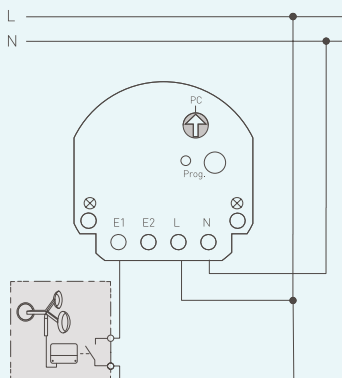
eNet universele zender en windsensor met 230 V-meldcontact
