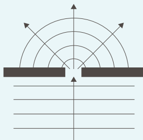
DiffRACTIE van elektromagnetische straling
