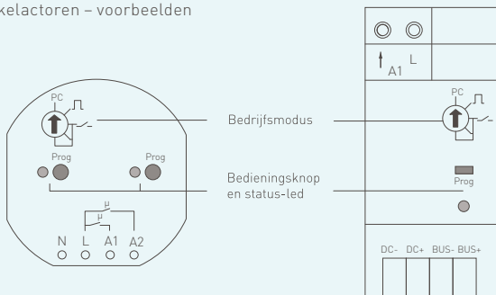
Schakelactoren – voorbeelden
