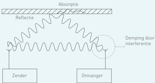
Demping en versterking van radiosignalen door interferentie
