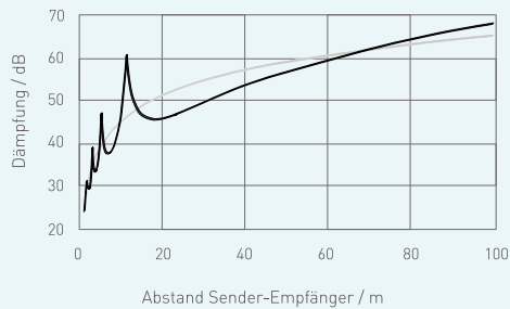
Dämpfung im Freifeld und im freien Raum
