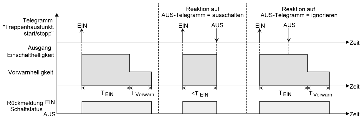
Bild 18: Ausschaltverhalten der Treppenhausfunktion ohne Soft-Funktionen
