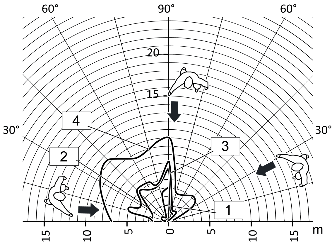
Rysunek 14: Zasięg przy promieniowym kierunku ruchu
