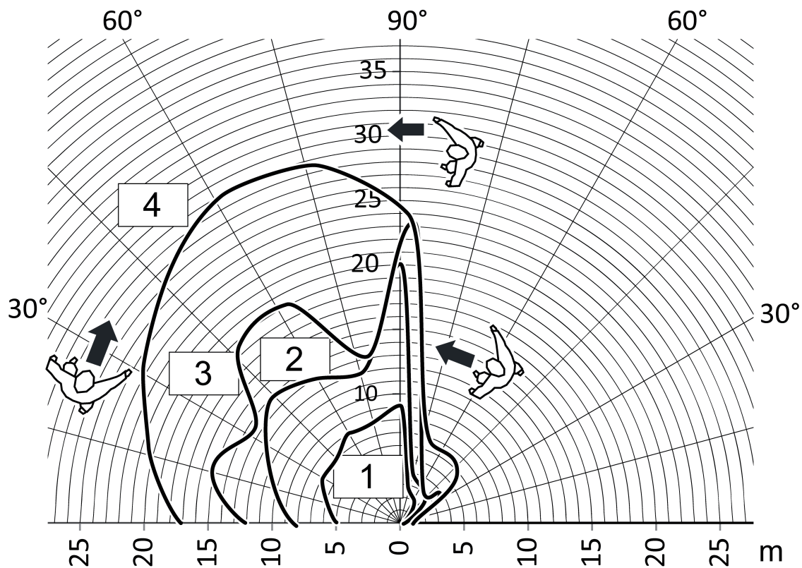
Rysunek 13: Zasięg przy styczonym kierunku ruchu
