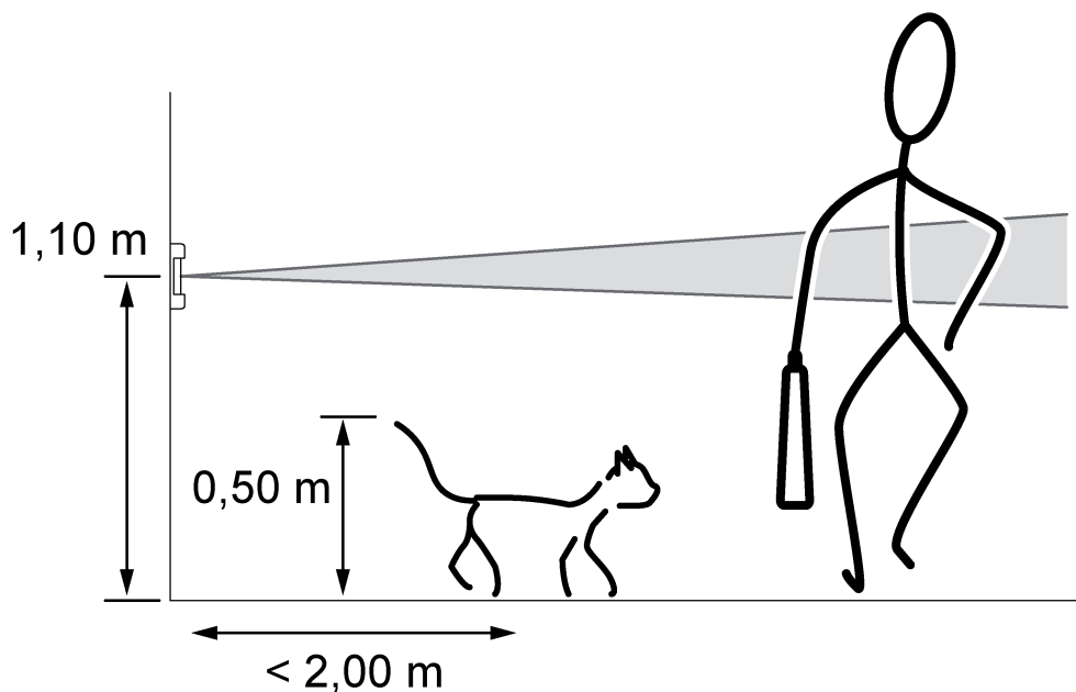
Rysunek 11: Pole widzenia i wysokość montażu
