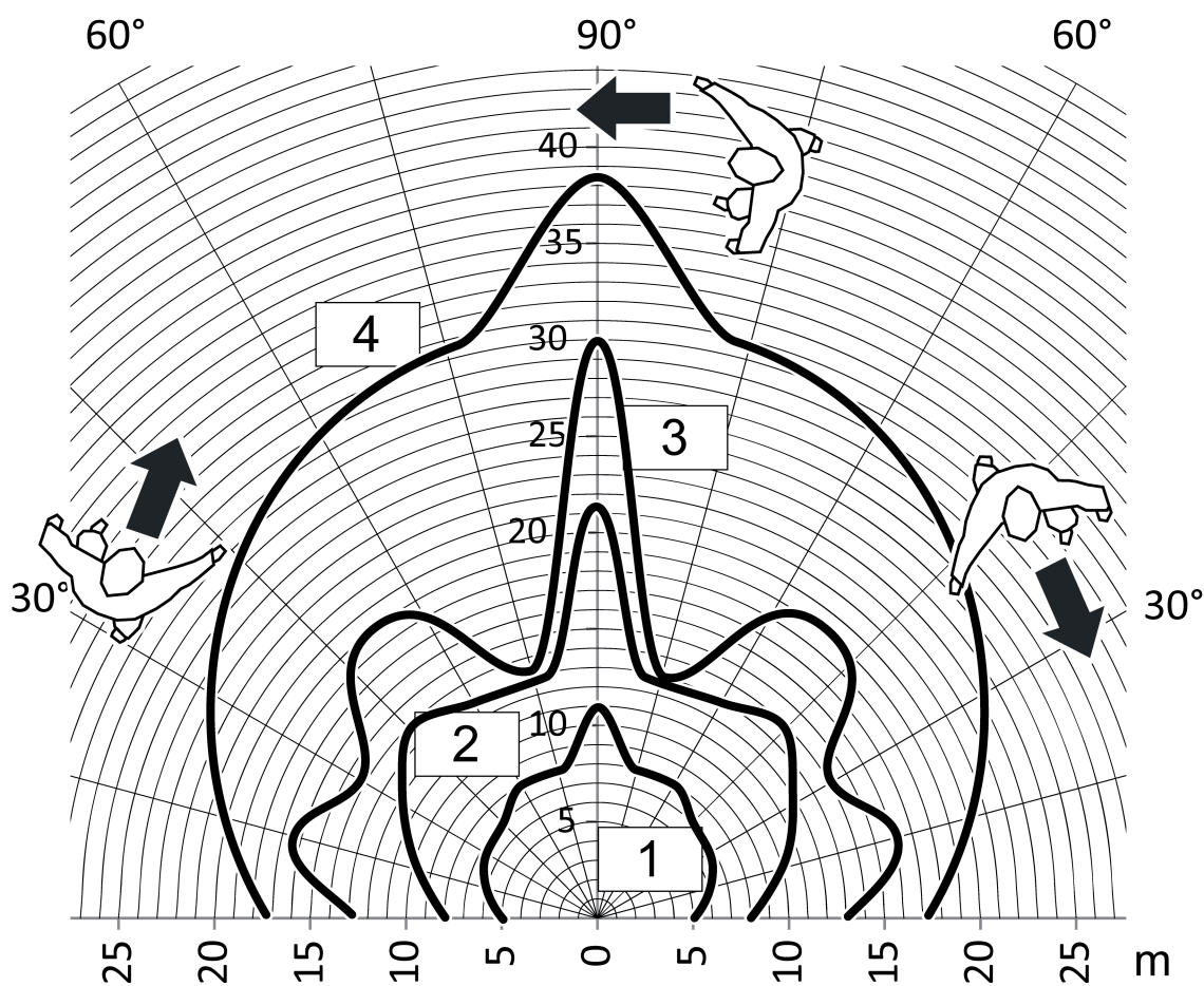
Rysunek 9: Zasięg przy styczonym kierunku ruchu
