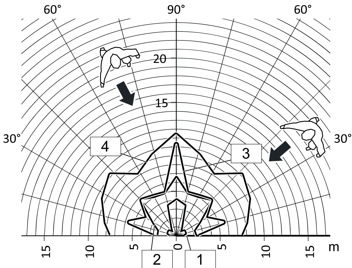
Rysunek 10: Zasięg przy promieniowym kierunku ruchu
