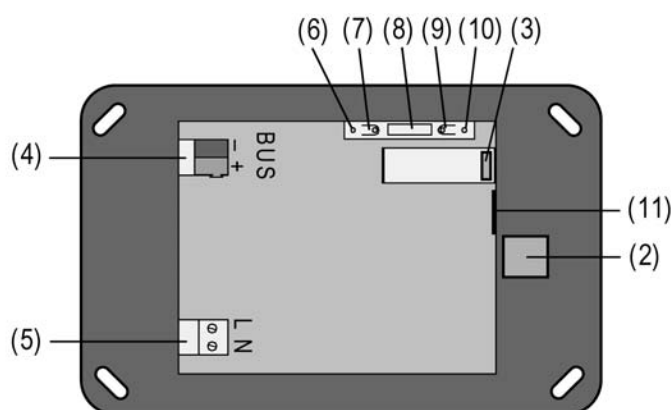
Bild 2: Geräteaufbau Rückseite
