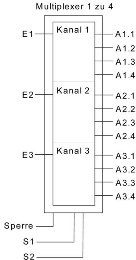
Bild 30: Multiplexer "1 zu 4"
