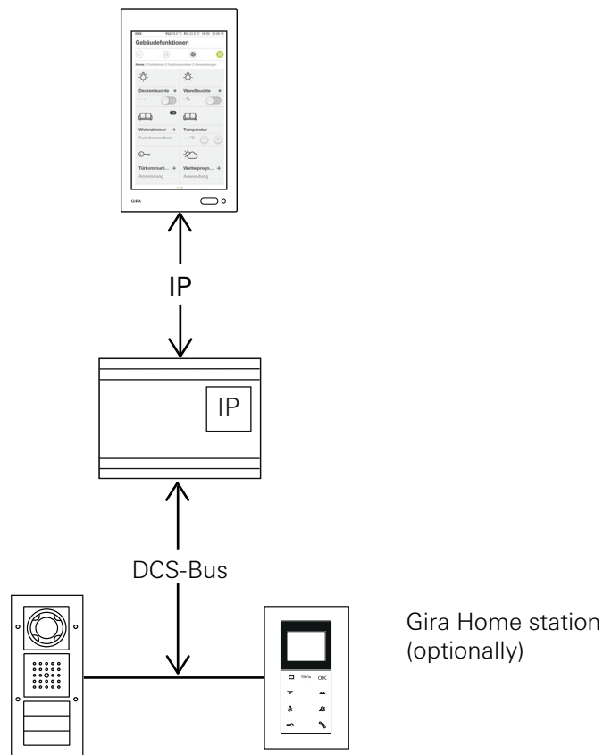
Bild 117 Gira G1 met DCS-IP-gateway.
