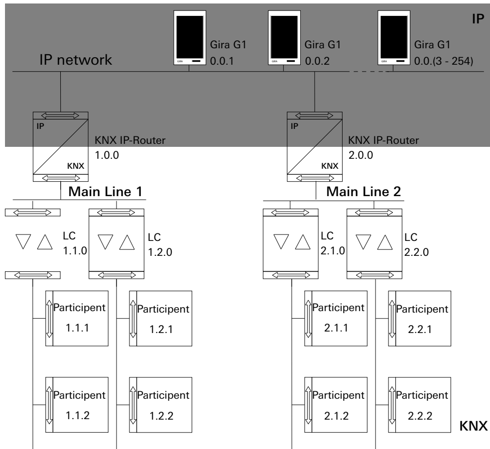
Bild 3 Voorbeeldtopologie: Gira G1 in Zonelijn
