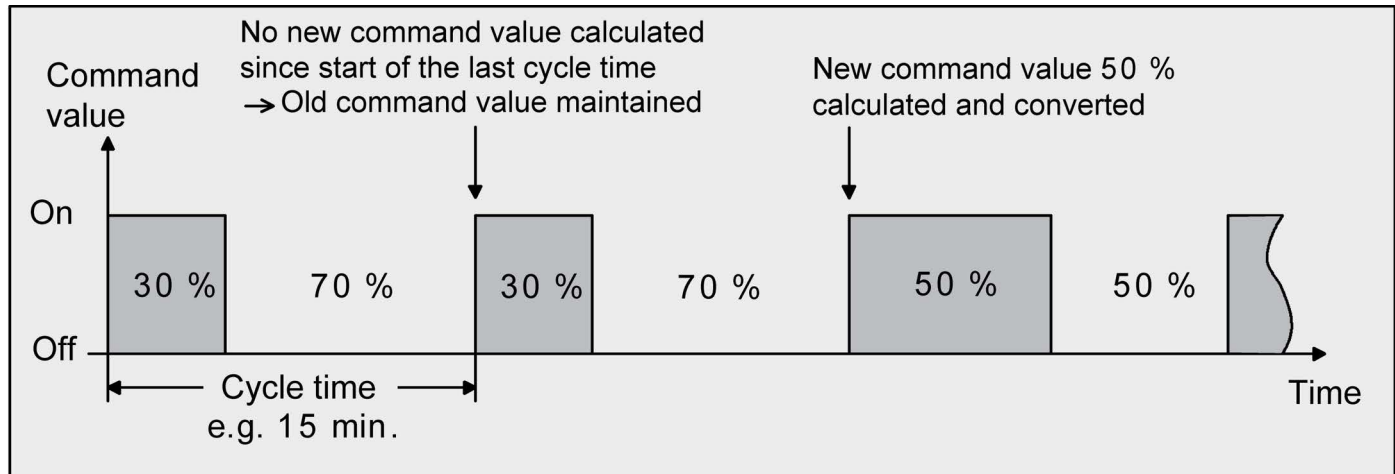
Bild 33: Switching PI control
