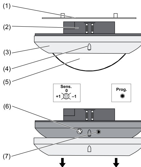
Figure 1: Conception de l'appareillage
