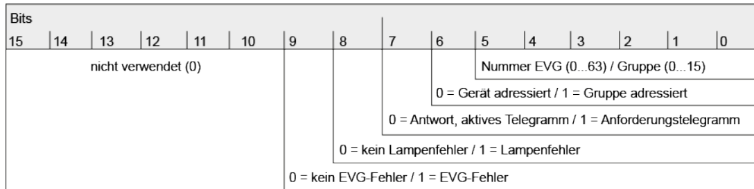
Bild 15: Telegrammaufbau 2-Byte-Fehlerstatus
