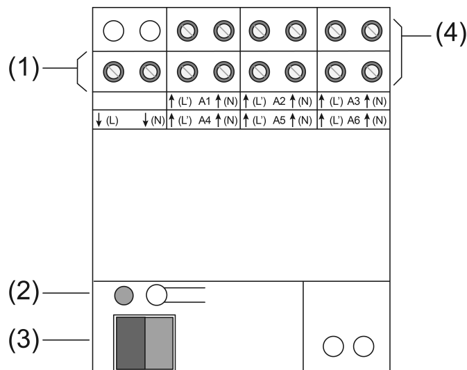
Figura 1: Vista frontale
