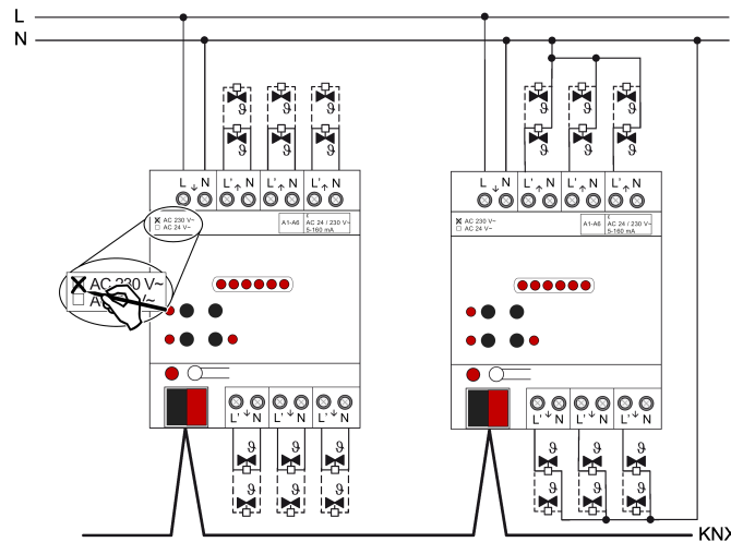
Figura 3: Conexión para accionamientos reguladores AC 230 V (ejemplos de conexión) izquierda: conductor neutro de los accionamientos reguladores guiados de forma independiente al actuador / derecha: conductor neutro común para accionamientos reguladores
