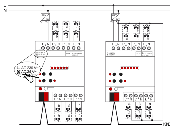
Figura 4: Conexión para accionamientos reguladores AC 24 V izquierda: conexión independiente de los accionamientos reguladores en el actuador / derecha: conductor común para accionamientos reguladores
