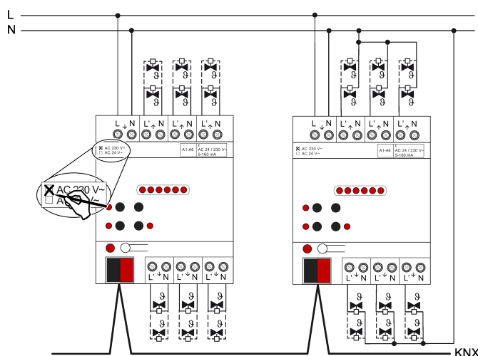
рисунок 3: Подключение сервоприводов 230 В перем. тока (примеры подключения)
