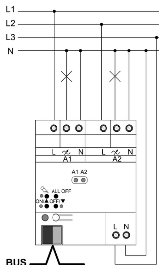
Afbeelding 4: Dimactor – Aansluitvoorbeeld
