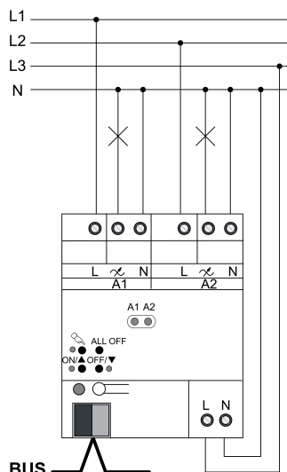
Rysunek 4: Ściemniacz – przykład podłączenia
