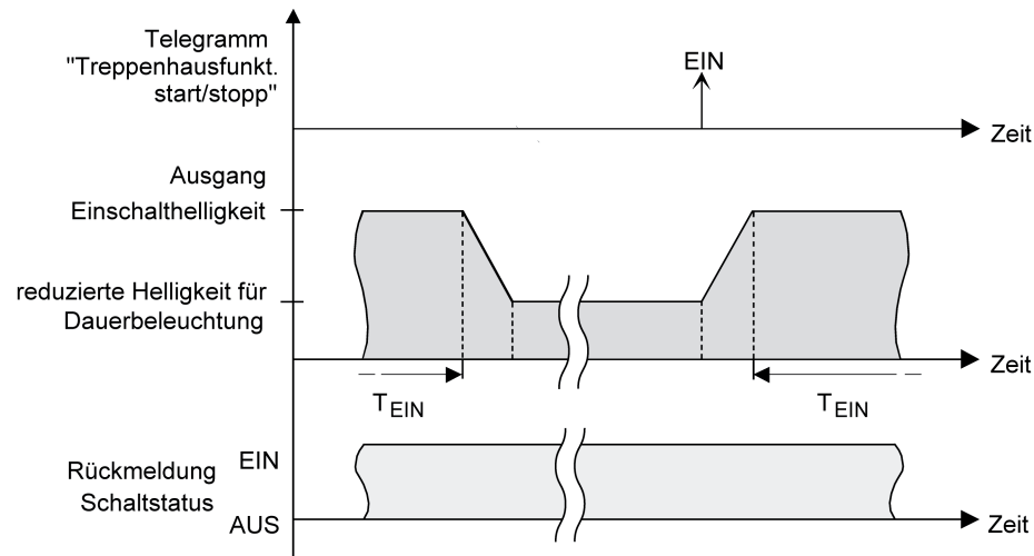
Bild 29: Die Dauerbeleuchtung der Treppenhausfunktion mit Soft-AUS-Funktion
