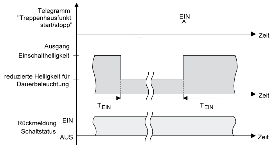
Bild 28: Die Dauerbeleuchtung der Treppenhausefunktion ohne Soft-Funktionen
