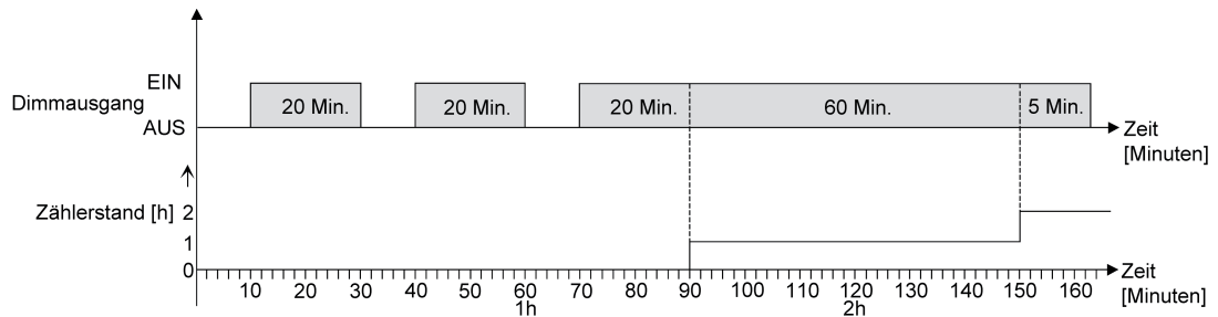
Bild 32: Funktionsweise des Betriebsstundenzählers (am Beispiel eines Vorwärtszählers)
