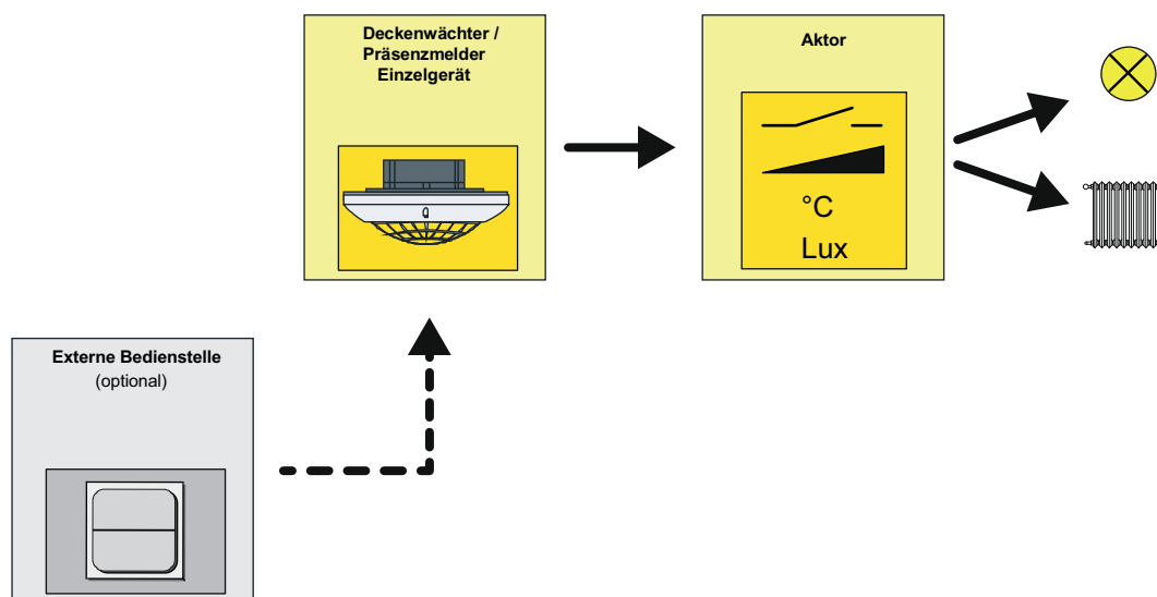
Bild 26: Applikationstyp "Einzelgerät"
