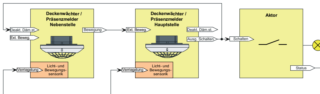
Bild 33: Applikationsbeispiel mit Dämmerungsstufenauswertung in der Hauptstelle und in den Nebenstellen für das Datenformat "Schalten"
