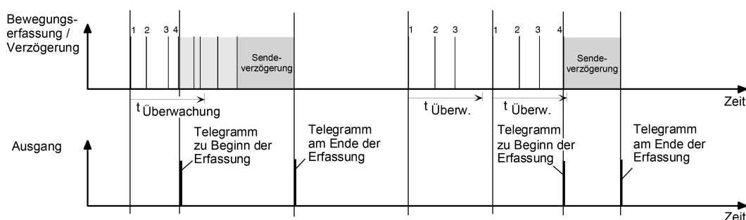
Bild 42: Bewegungsauswertung beim Melder
