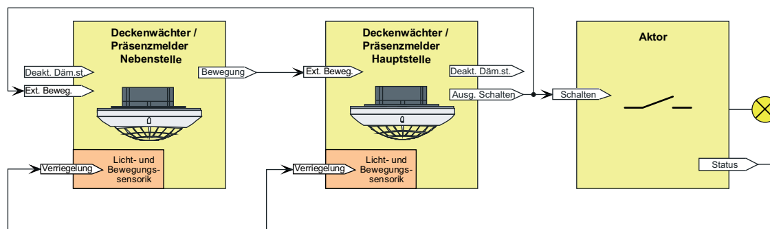
Bild 35: Applikationsbeispiel mit Dämmerungsstufenauswertung in der Hauptstelle und in den Nebenstellen für Ausgangsfunktion "Treppenhausfunktion"
