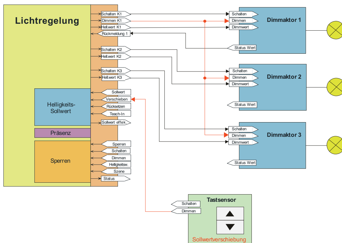
Bild 49: Applikationsbeispiel zur Sollwertverschiebung mit 3 Beleuchtungskanälen
