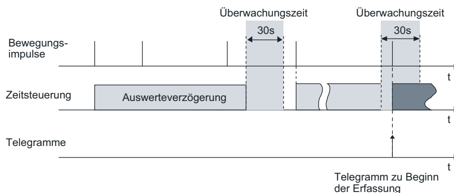
Bild 41: Auswertverzögerung mit nur kurzzeitiger Bewegung
