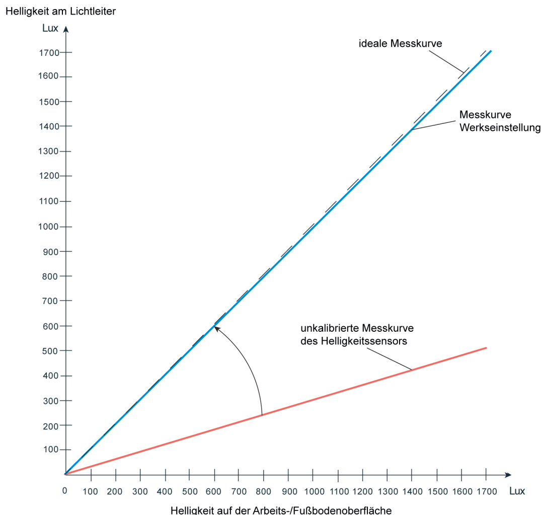
Bild 18: Bestimmung der Helligkeit an der Arbeits- / Fußbodenoberfläche bei Werkseinstellung Reflexionsfaktor 0,3 entspricht Oberflächenbeschaffenheit (graue Schreibtischoberfläche)
