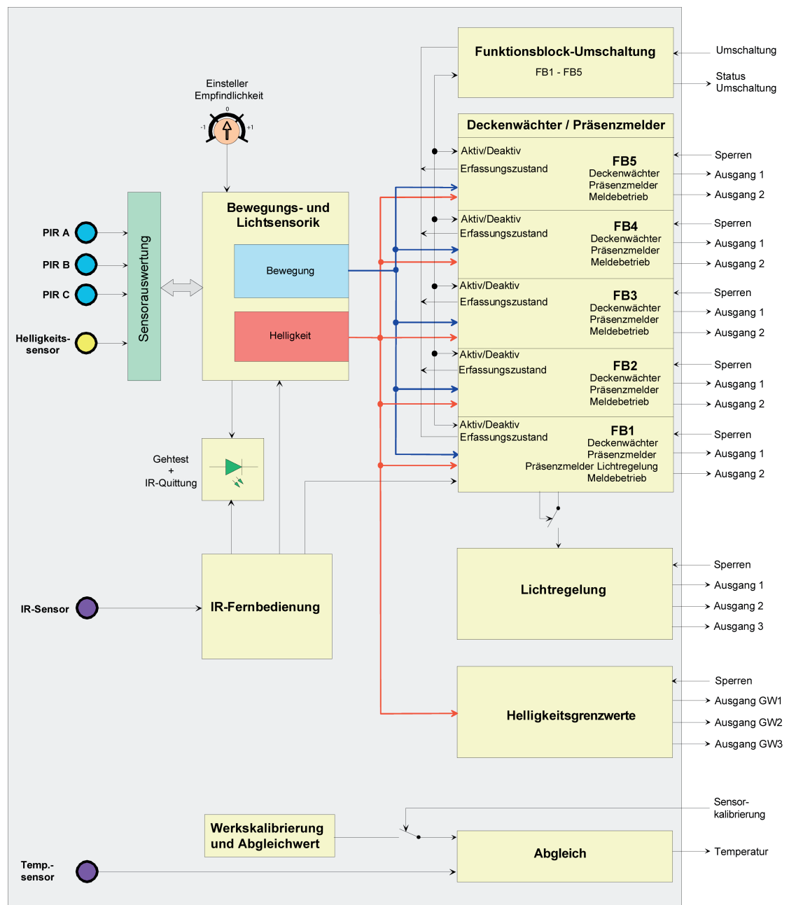
Bild 15: Blockschaltbild aller Funktionen des Geräts
