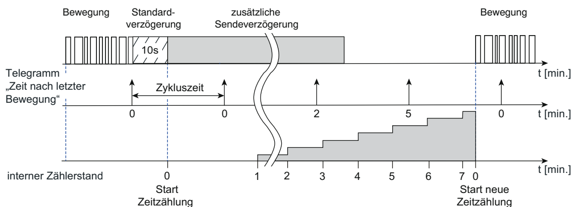
Bild 43: Messung der Zeitspanne nach letzter Bewegung
