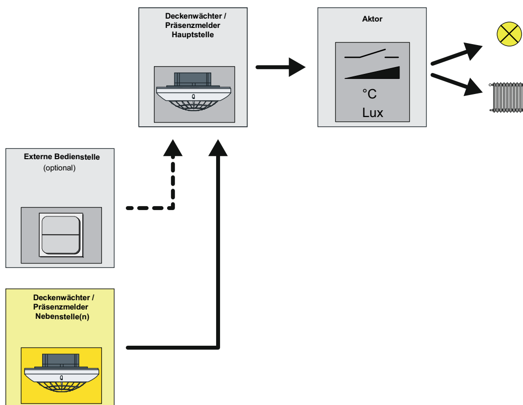
Bild 28: Applikationstyp "Nebenstelle"
