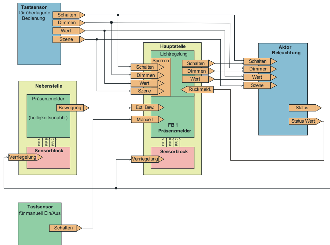
Bild 61: Applikationsbeispiel 1
