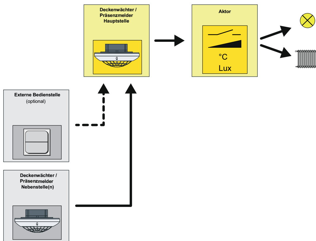
Bild 27: Applikationstyp "Hauptstelle"
