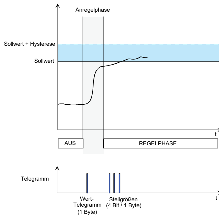
Bild 55: Anregelverhalten mit absoluten Wert-Telegrammen (1 Byte)
