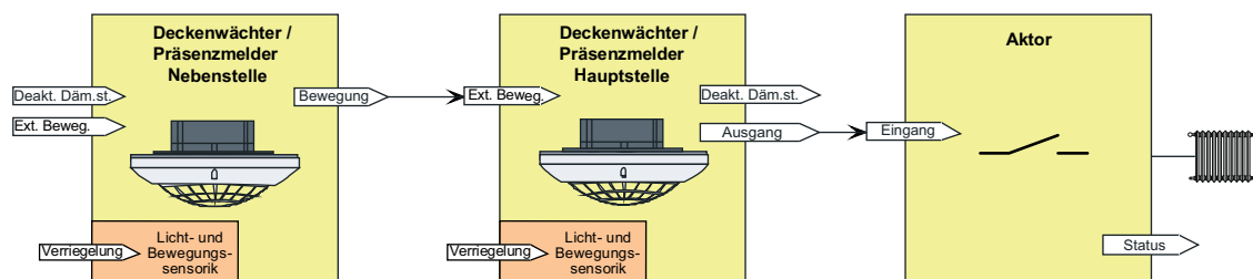
Bild 36: Applikationsbeispiel ohne Dämmerungsstufenauswertung in der Hauptstelle und in den Nebenstellen
