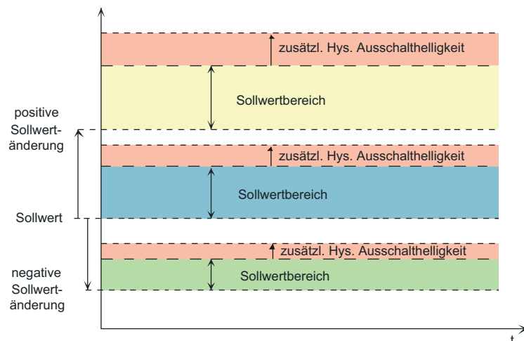
Bild 59: Abhängigkeit der zusätzlichen Hysterese für die Ausschalthelligkeit bei einer Sollwertverschiebung
