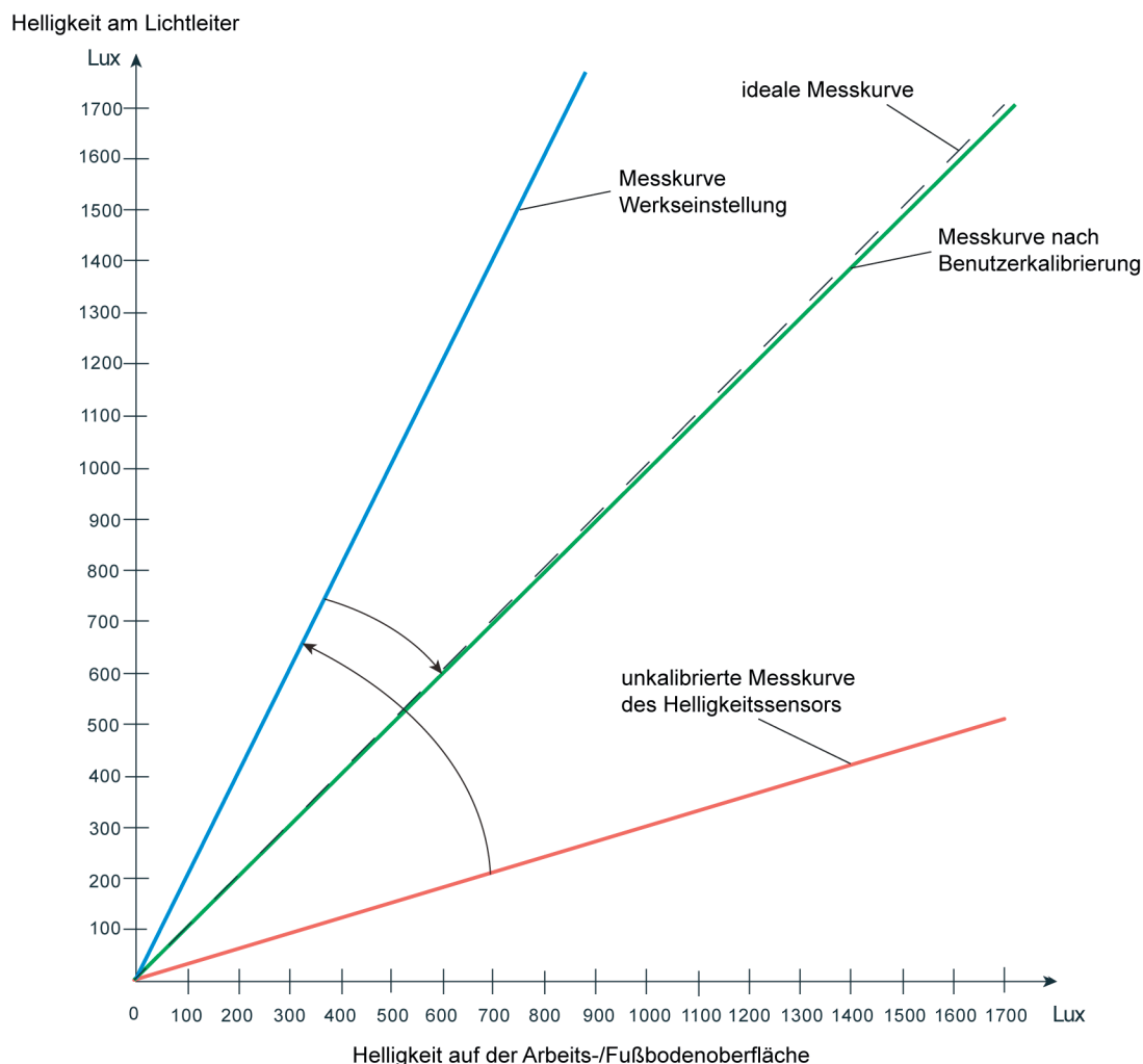
Bild 19: Korrektur der ermittelten Helligkeit an der Arbeits- / Fußbodenoberfläche durch Benutzerkalibrierung z. B. Reflexionsfaktor 0,5 entspricht Oberflächenbeschaffenheit (heller Fußbodenbelag)
