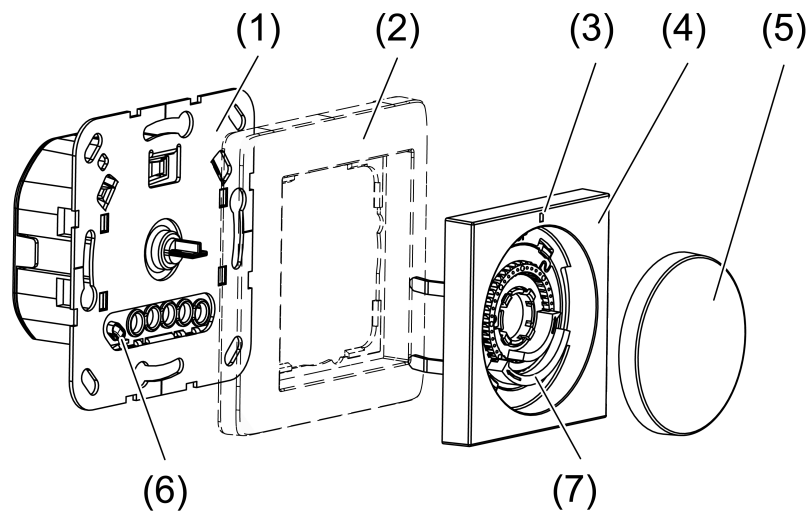
Bild 1: Geräteaufbau
