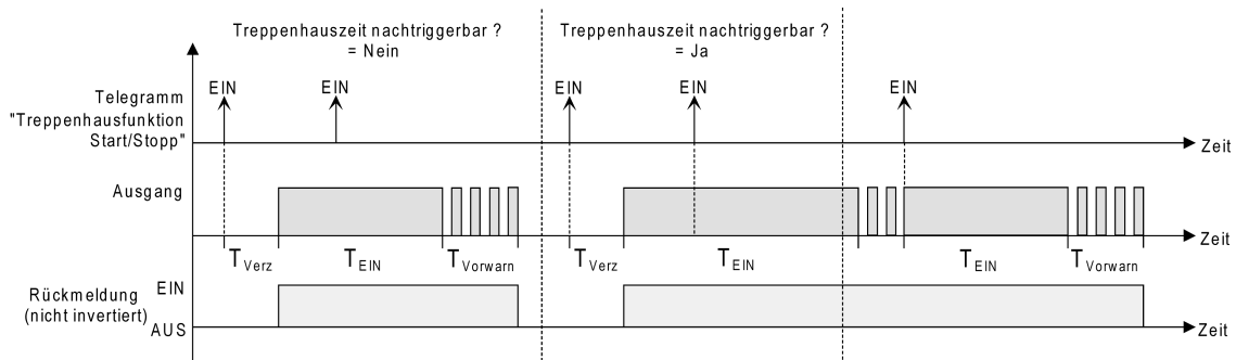
Bild 19: Einschaltverhalten der Treppenhausfunktion
