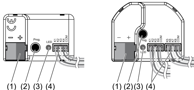
Afbeelding 1: Constructie apparaat
