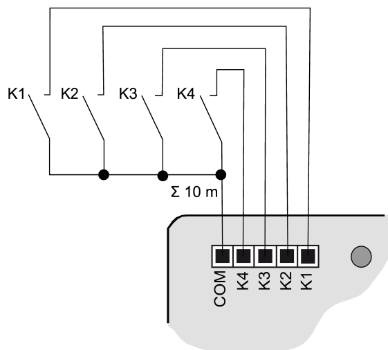
Afbeelding 3: Aansluitvoorbeeld 4-voudig
