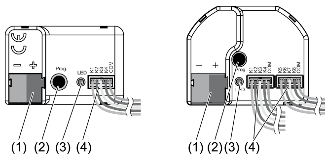
rysunek 1: Budowa urządzenia
