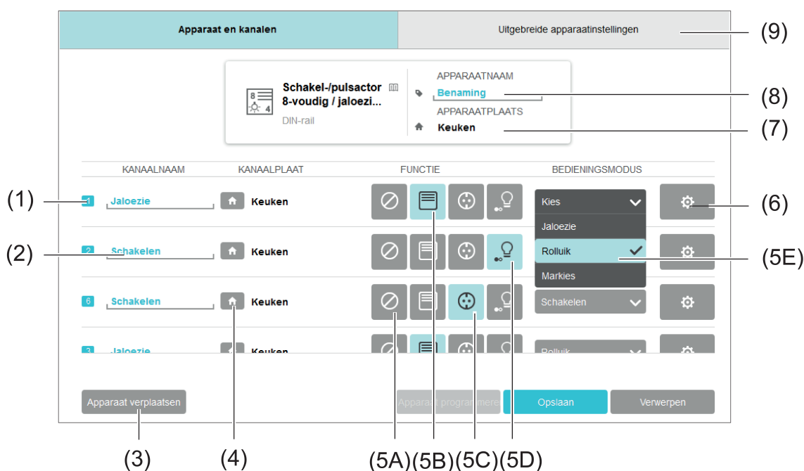
Afbeelding 12: Venster Apparaatinstellingen - voorbeeld schakel-/jaloezieactor
