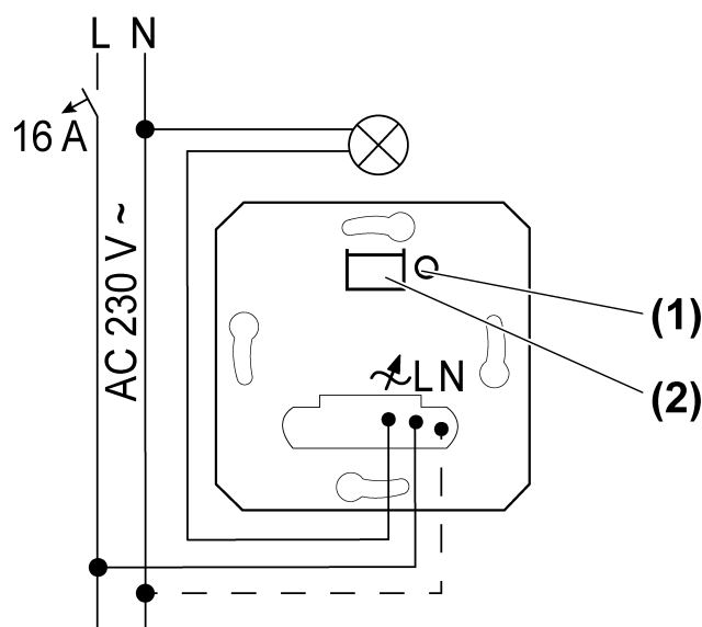
Imagem 1: Esquema de ligações
