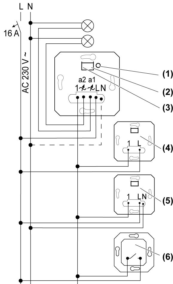
Afbeelding 1: Aansluitschema met optionele nevenaansluitingen
