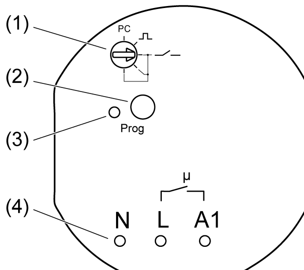
Afbeelding 1: Radiografische schakel-/pulsactor
