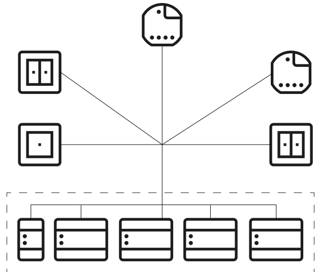
Câblage en étoile
