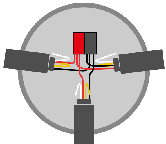
Raccordement des participants au bus
