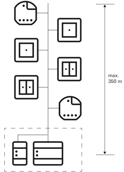
Distance alimentation – participants : 350 m max.
