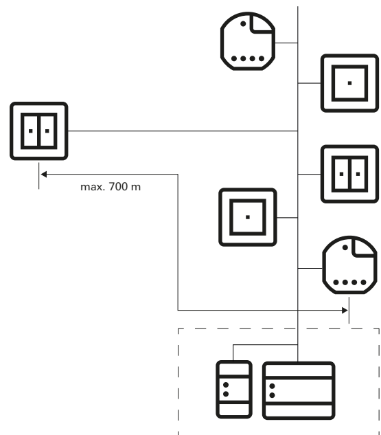
Distance entre deux participants quelconques : 700 m max.
